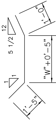
#3 BARS M N.T.S.
