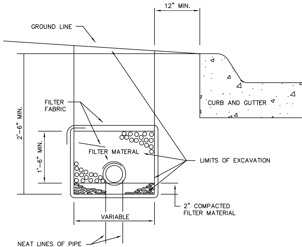
SECTION N.T.S.
